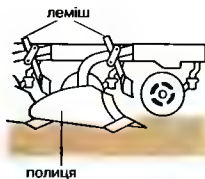
Плуг Перша секція багатоскибового плуга
